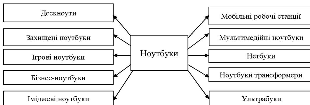
Рис. 1. Класифікація ноутбуків
